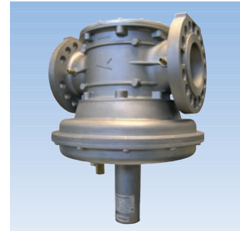
Tipo/Type VRGA
