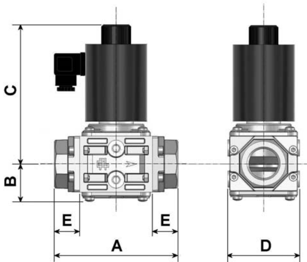
Tipo/Type AMSV..5R
